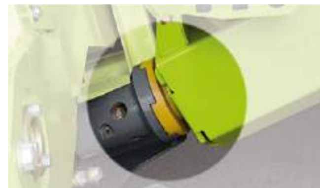
Trasmissione della potenza tramite attacco rapido.
