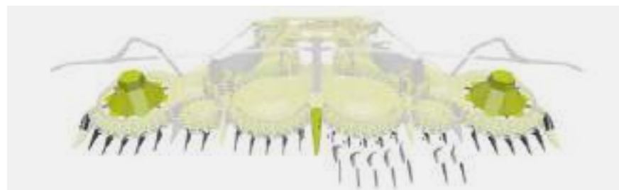
Coni coclee per mais allettato, elementi convogliatori ed estensioni delle punte come equipaggiamento supplementare.
